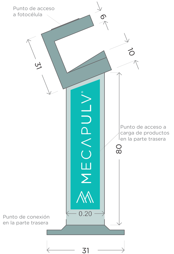
ALZADO LATERAL
